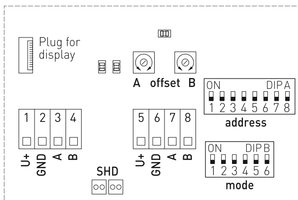
Схема подключения
