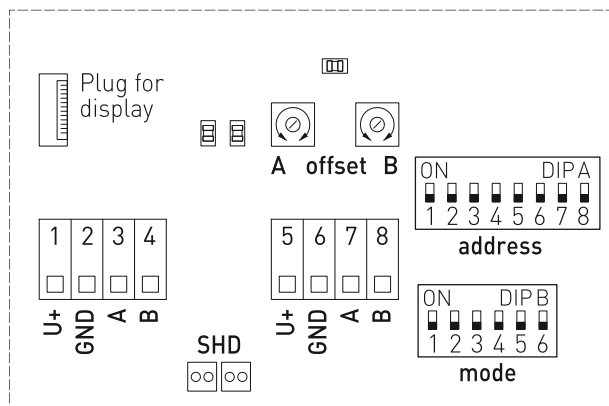
Schéma de raccordement
